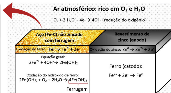
Figura 2: Representação esquemática de reações químicas e eletroquímicas que ocorrem em uma peça metálica, tendo uma região revestida com zinco e outra região sem proteção exibindo produtos de corrosão (ferrugem).
